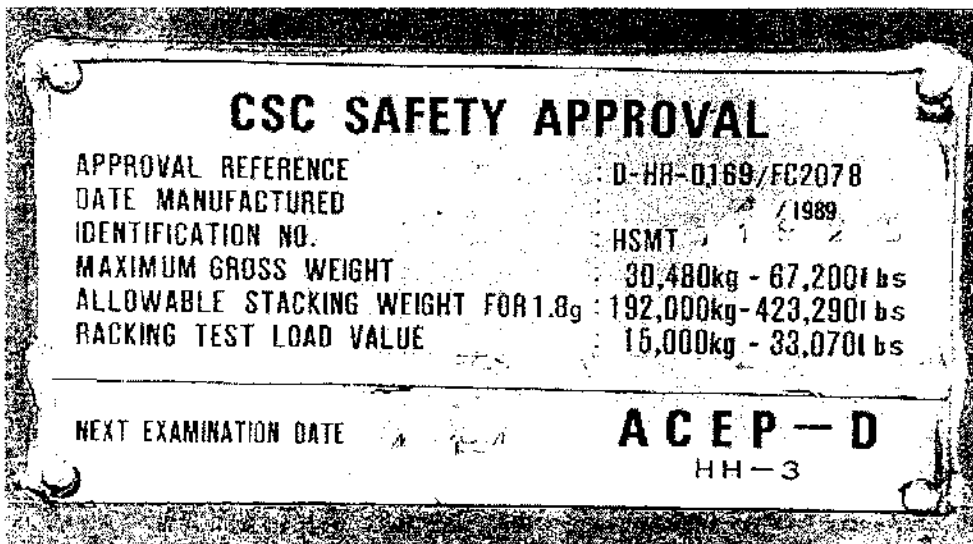
Abbildung 6: CSC-Plakette (Hapag-Lloyd AG, Hamburg, [46])
